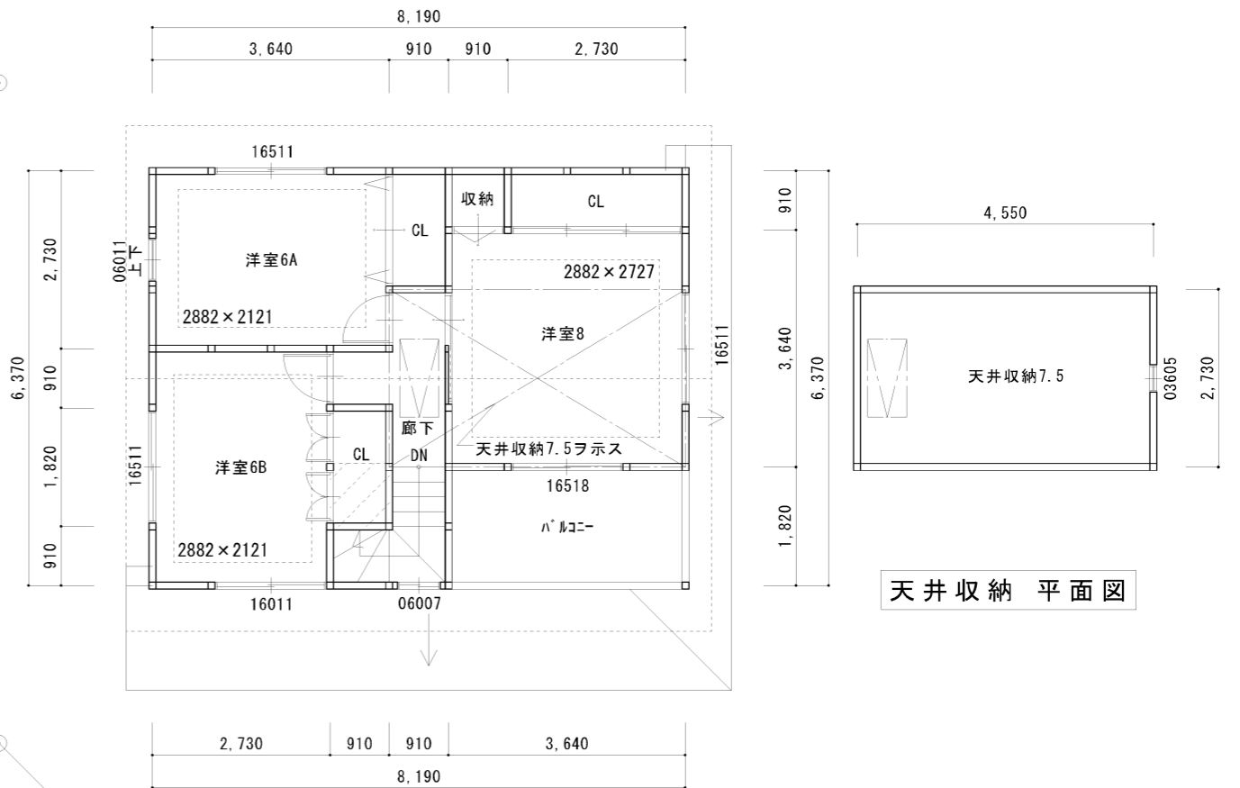
2階 平面図 45.55m 2
