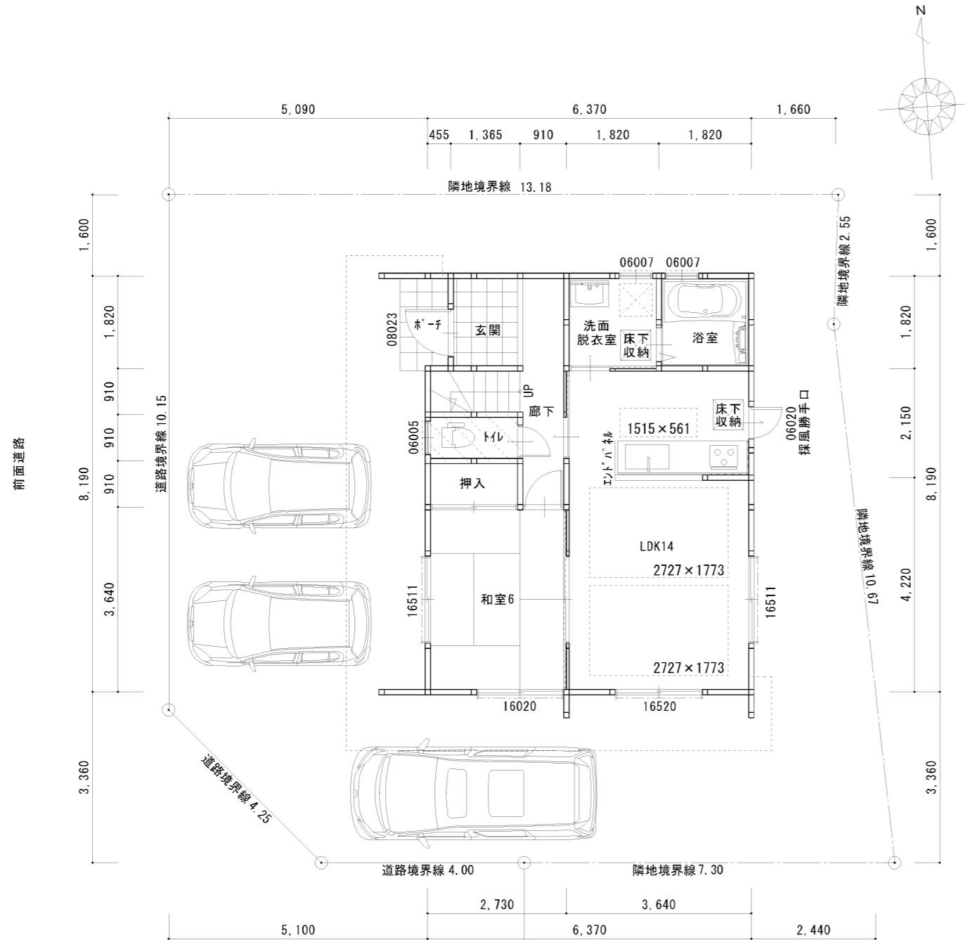
1階 平面図
