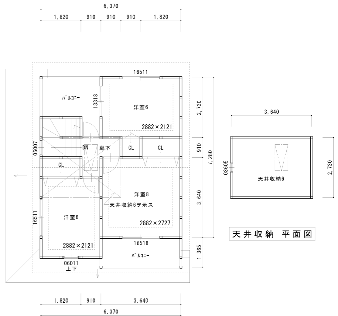
2階 平面図
